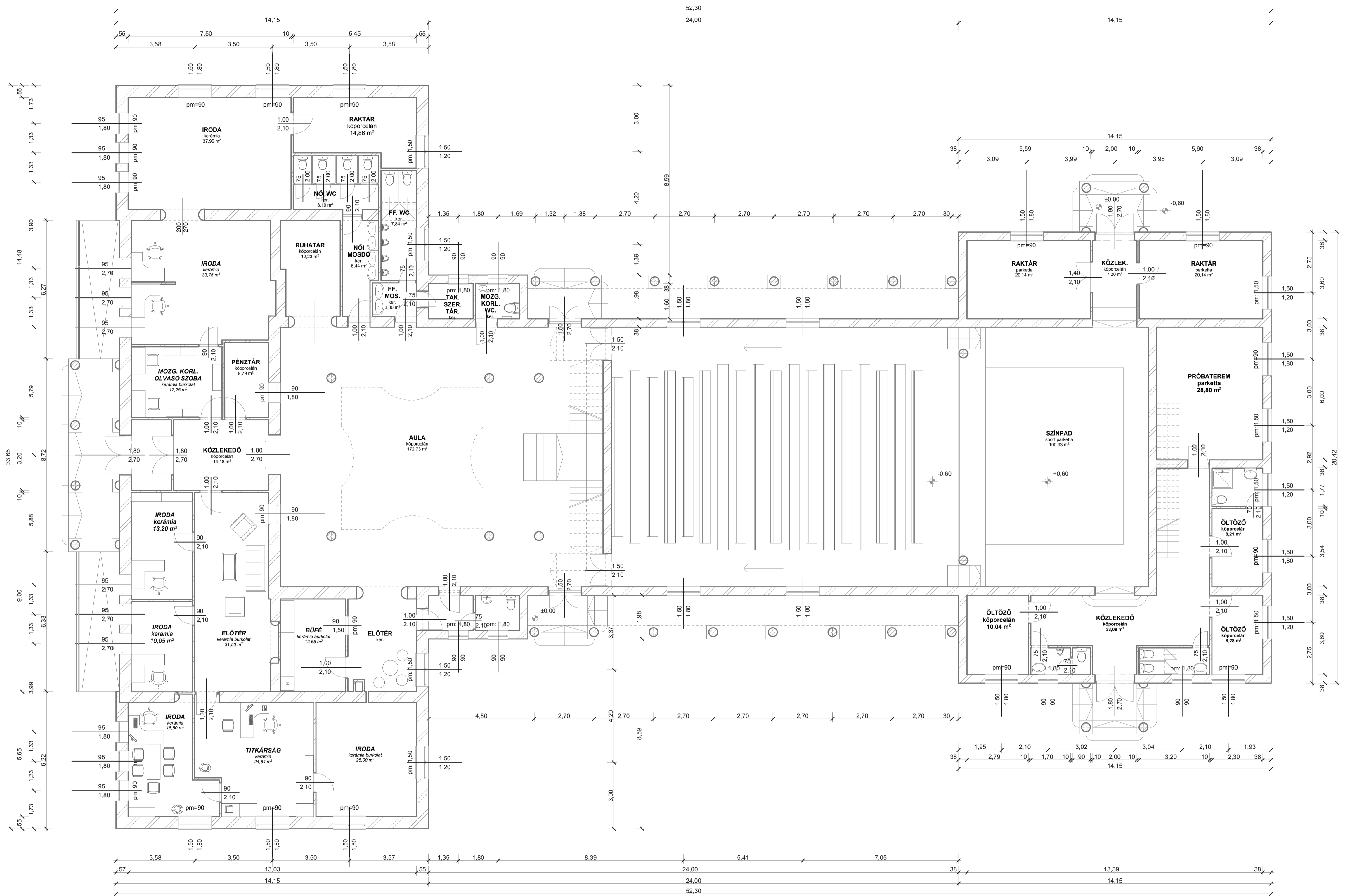
FÖLDSZINT FELMÉRÉSI ALAPRAJZ M=1:100
